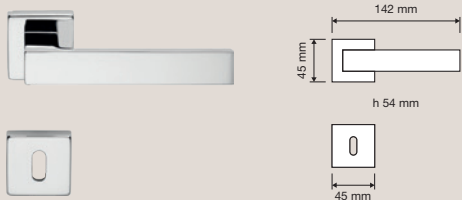
505 RB 014 Maniglia con rosetta art.014 / Door handle on rose art.014
